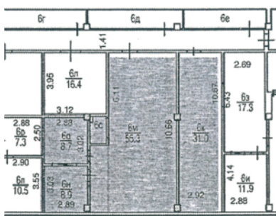
Планировка помещения
