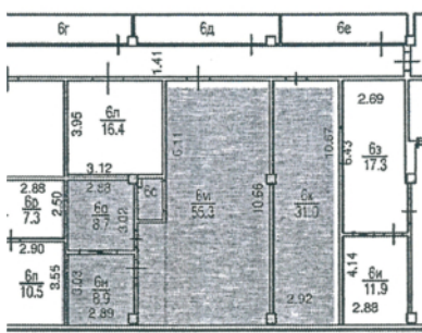
Планировка помещения
