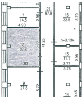
Планировка помещения
