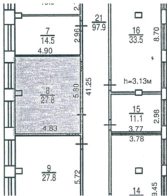
Планировка помещения
