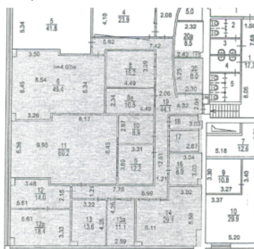
Планировка помещения
